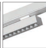
Afdekplaat (1482 mm) met 3-fase inbouwrail (683 mm) voor het integreren met 3-fase railsspots, bijv. ISS.1 DALI
