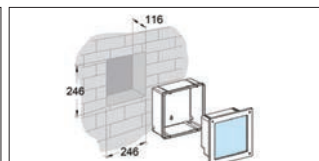
Inbouwdoos incl. (apart/vooraf leverbaar)
