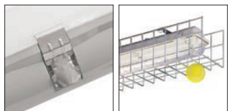
RVS kapklem (optie)
