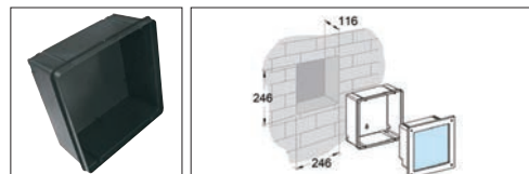
Inbouwdoos incl. (apart/vooraf leverbaar)
