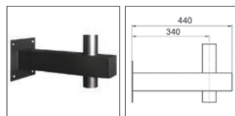
KGL.9200.35 Wanduihouder (optie)
