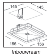
Inbouwraam
