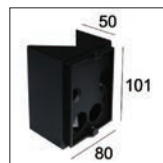
Wandhoeksteun (optie)
