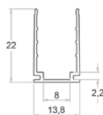
Aluminium profiel
