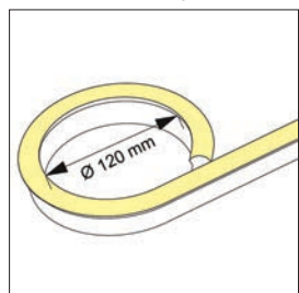
Horizontaal buigbaar
