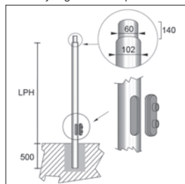
PSL.3 Conisch Ø 102
