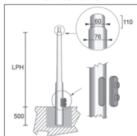
PSL.2 Verjongd / Verloop Ø 76
