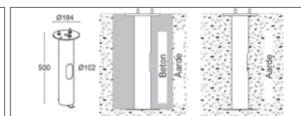
ARC.9220.00 Fundatie
