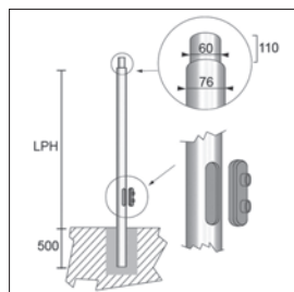
PSL.1 Conisch Ø 76
