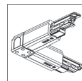
3FR.6350.xx XTSC 635 Hoekstuk 90° vast rechts
