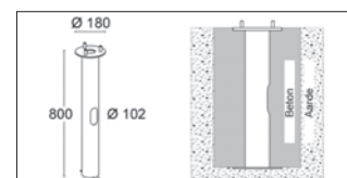
ARC.9230.00 Fundatie (optie)
